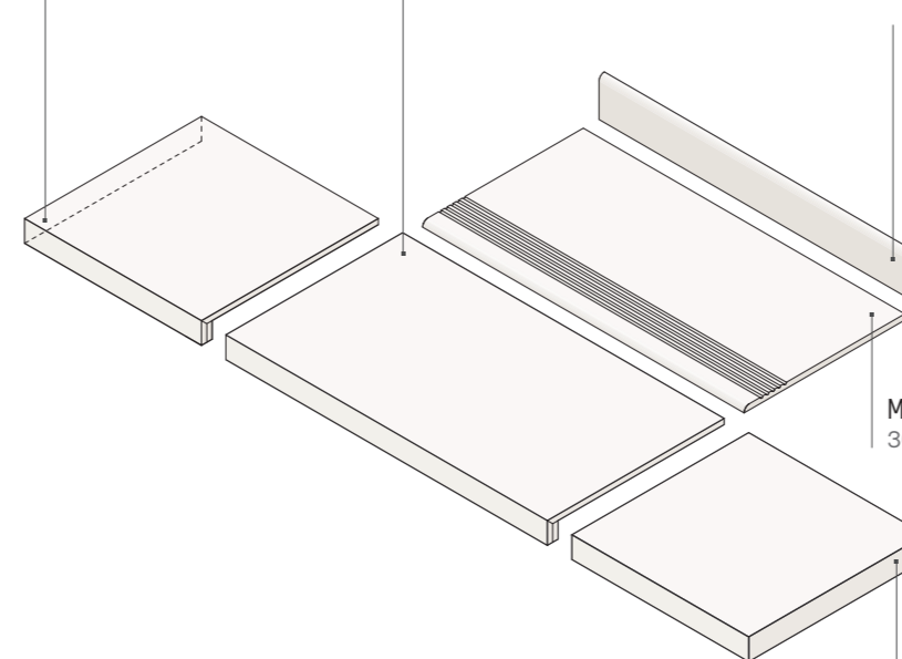
Marvel Scalino Angolare Sx ✓ 33x33 cm - 13"x13"
